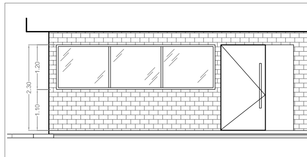
FACHADA SOBRE CONSTITUYENTES
