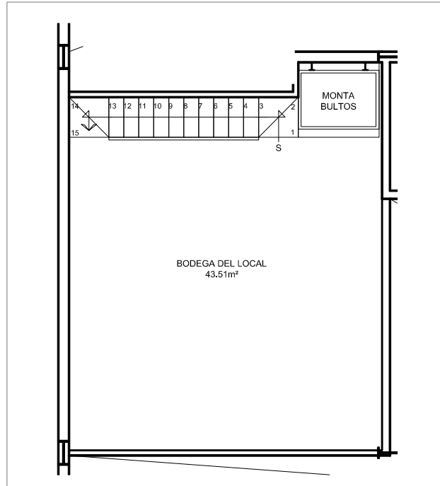
PLANTA DE BODEGA EN SÓTANO
