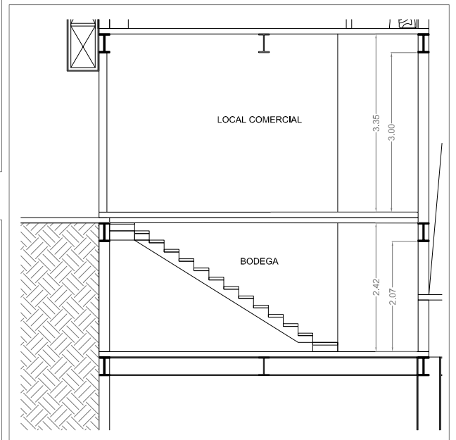
CORTE DEL LOCAL Y SU BODEGA
