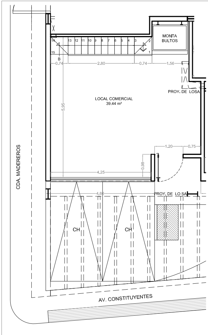
PLANTA BAJA
